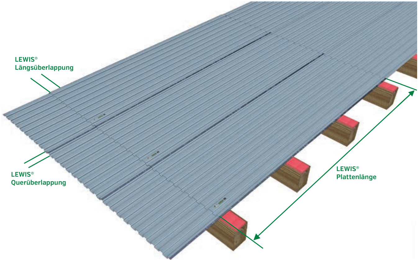
LEWIS®-Schwalbenschwanzplatten Verlegung
